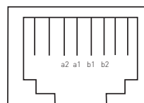
Belegung der internen S0s
