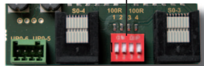
Abschlusswiderstände S0-3, S04
